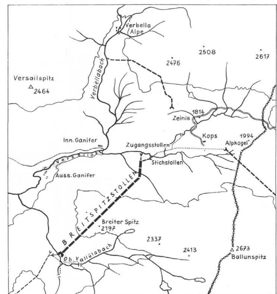
Lageplan des Breitspitzstollens (Ausschnitt aus Sektion 5244/1 u. 2)
